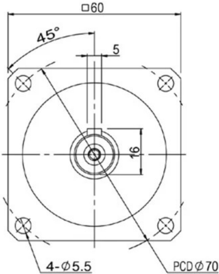
輸出端(output)
