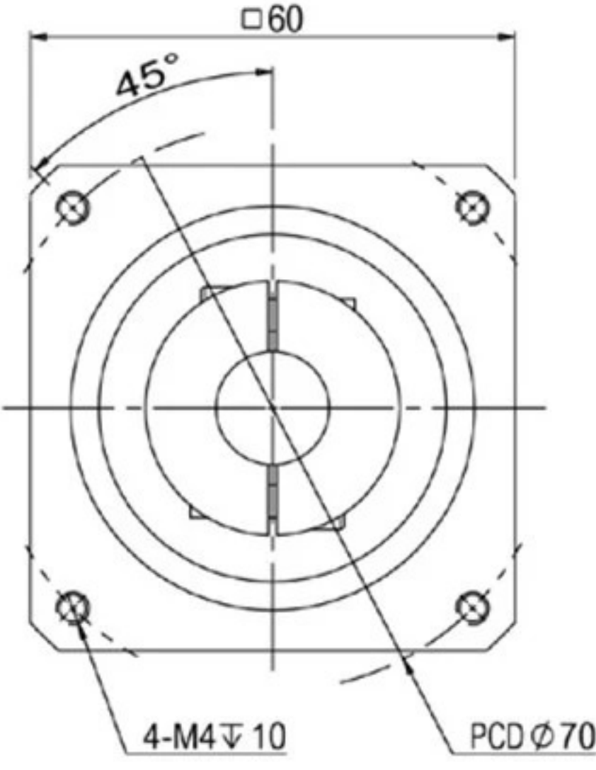
輸入端(input)
