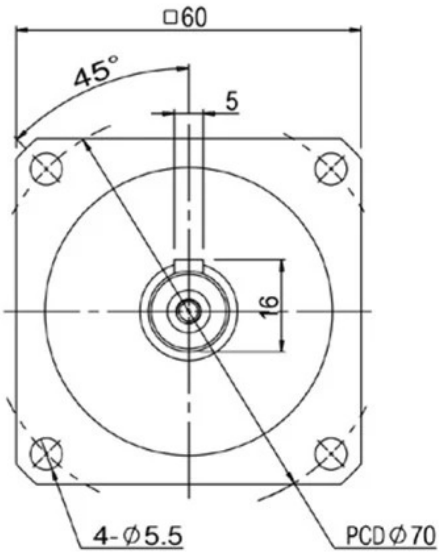
輸出端(output)
