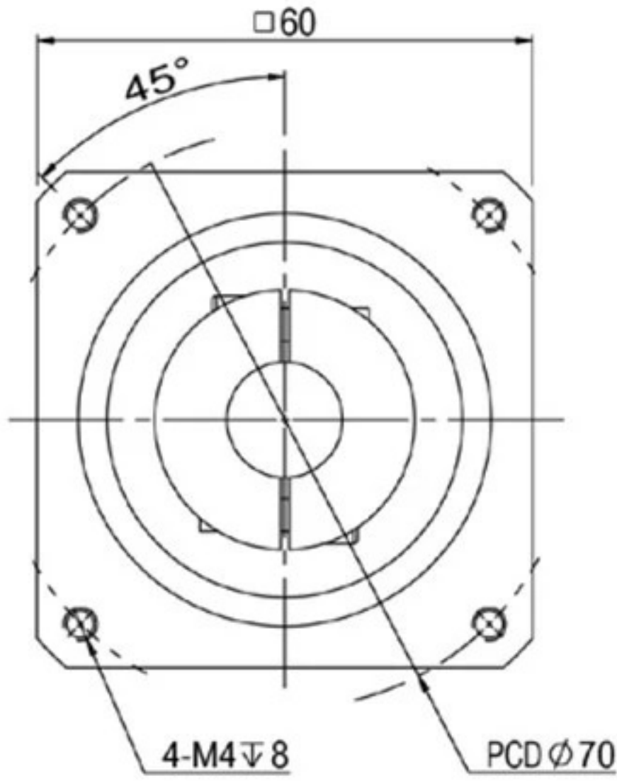
輸入端(input)
