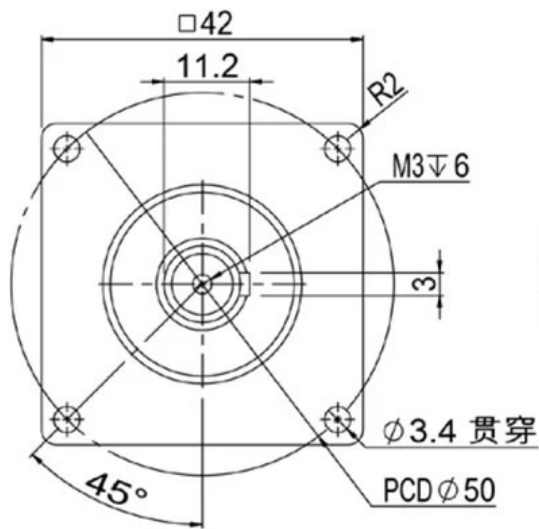
輸出端(output)
