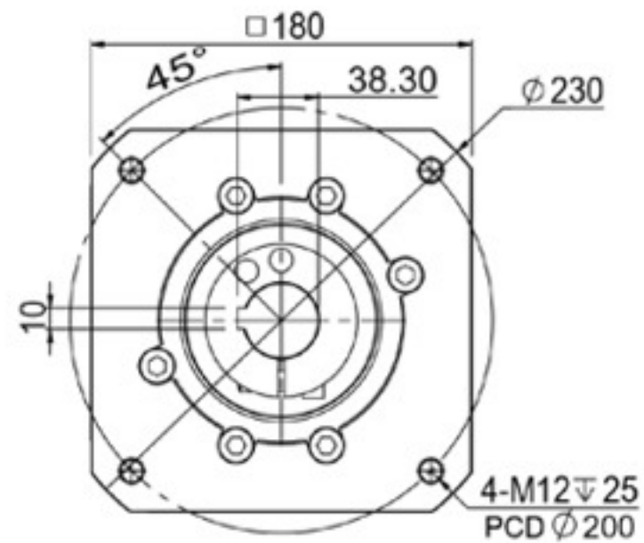
輸入端(input)
