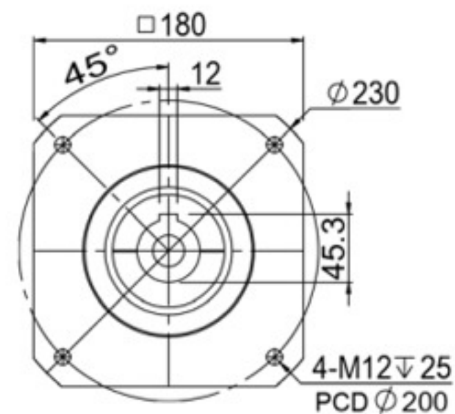
輸入端(input)
