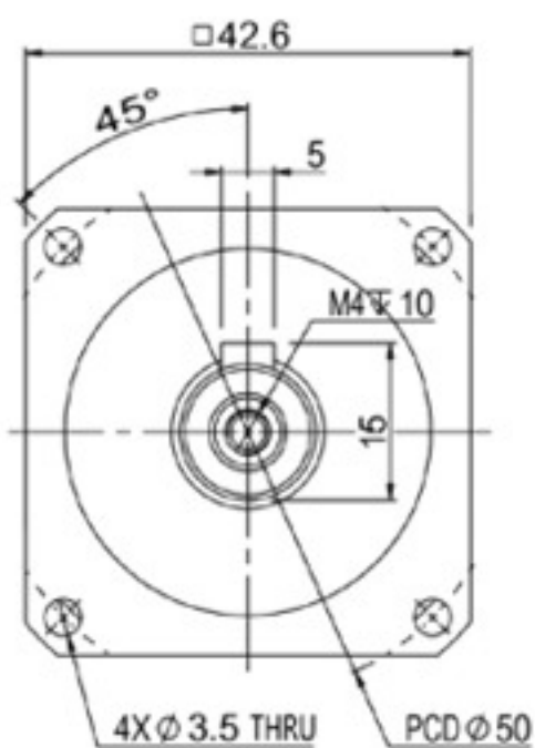
輸出端(output)
