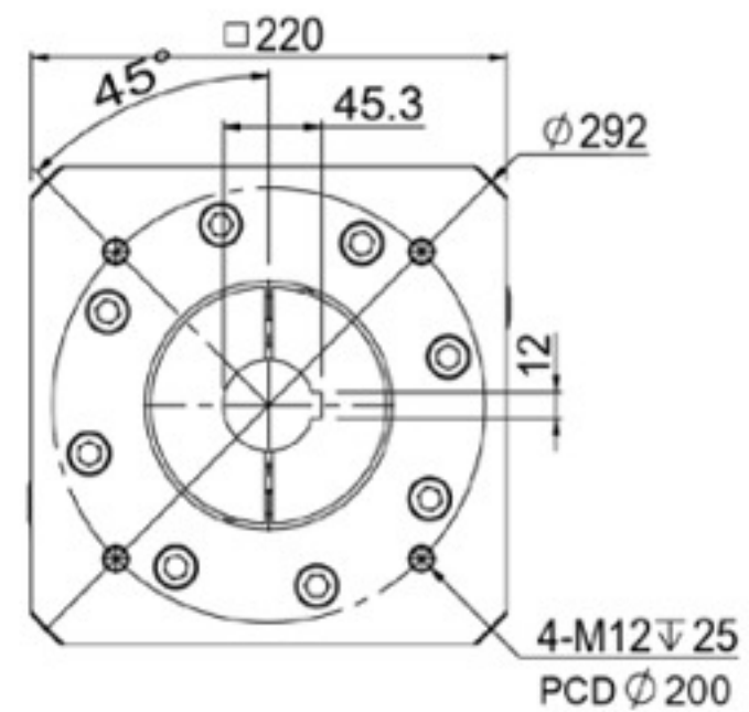
輸入端(input)
