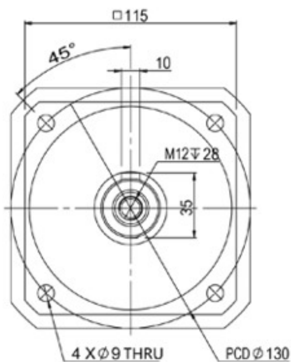
輸出端(output)
