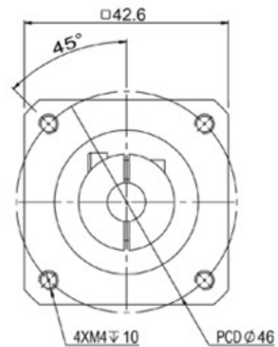
輸入端(input)
