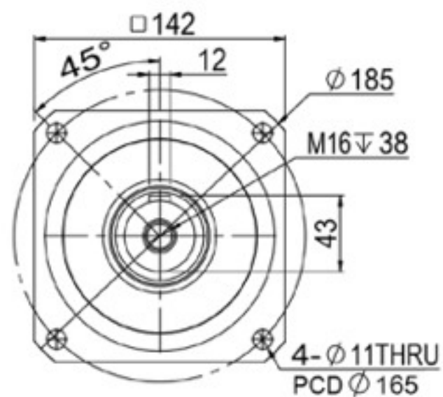
輸出端(output)
