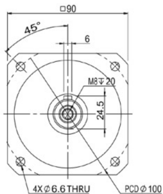
輸出端(output)
