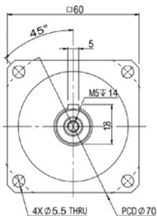
輸出端(output)
