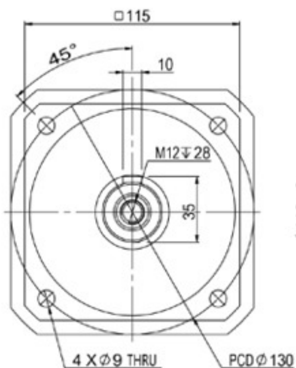
輸出端(output)
