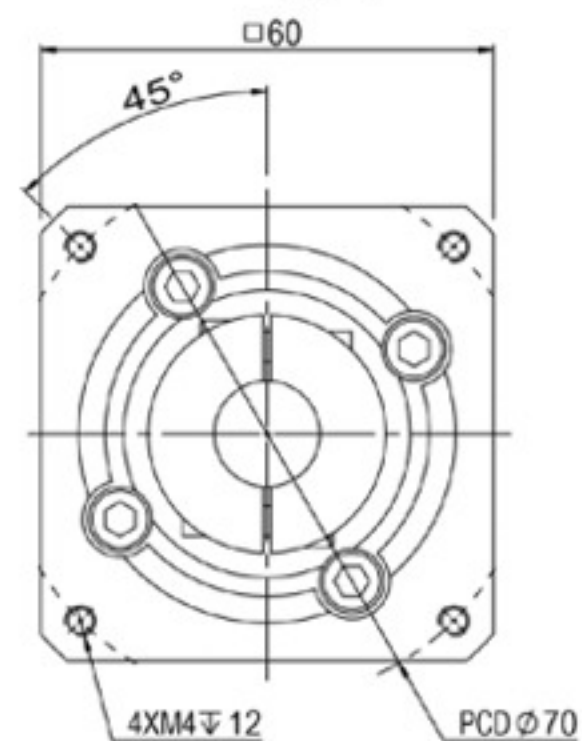
輸入端(input)
