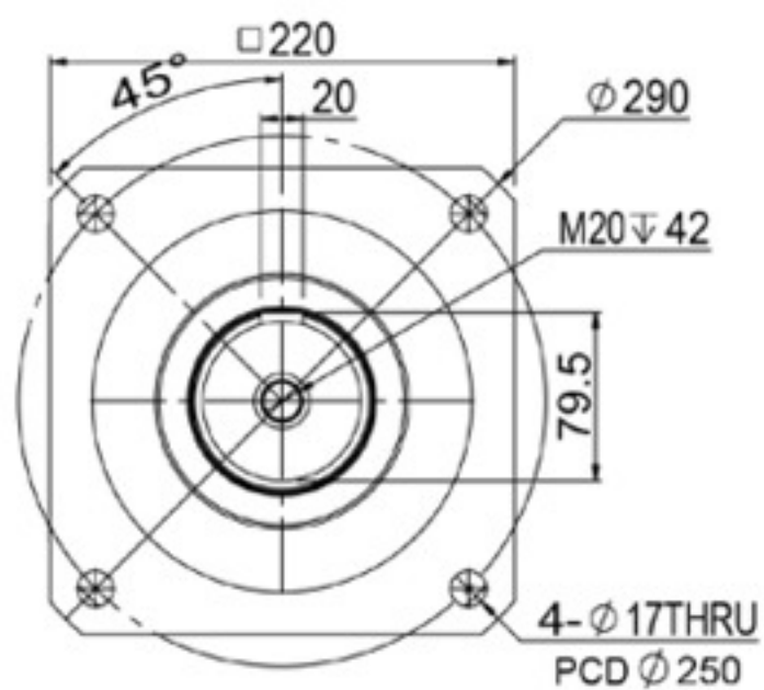
輸出端(output)
