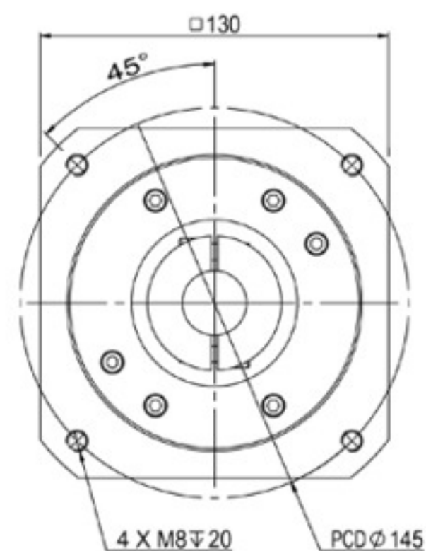
輸入端(input)
