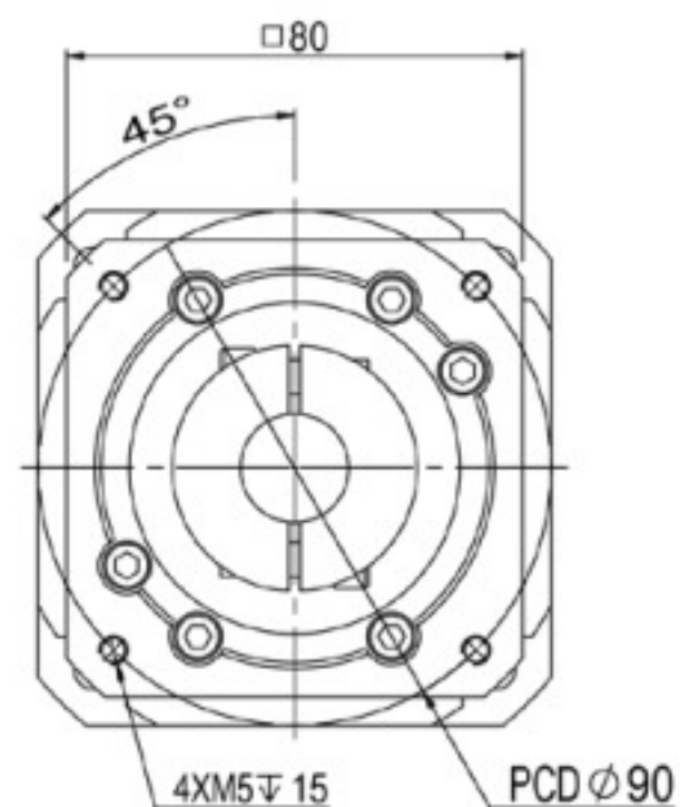
輸入端(input)
