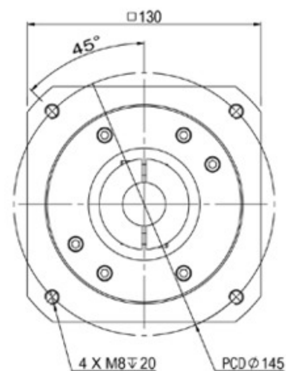
輸入端(input)
