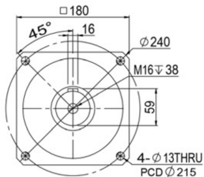
輸出端(output)
