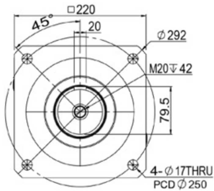
輸出端(output)
