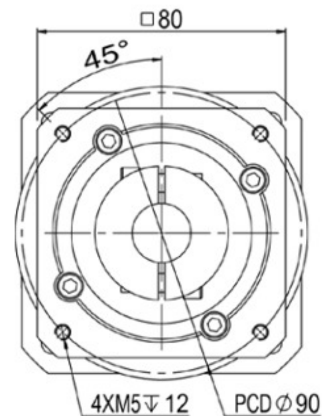
輸入端(input)
