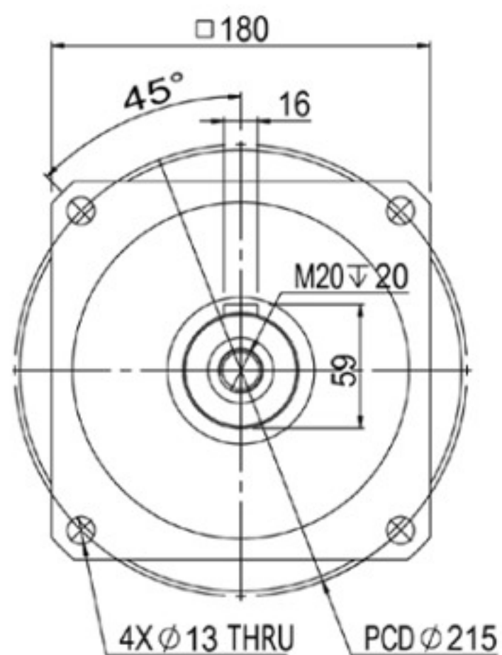
輸出端(output)
