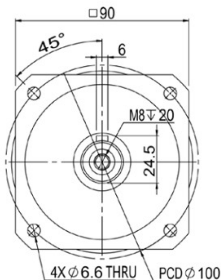
輸出端(output)
