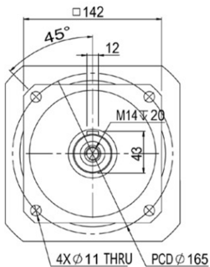
輸出端(output)
