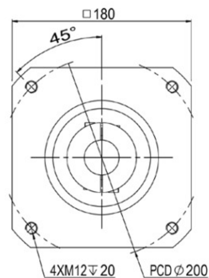
輸入端(input)
