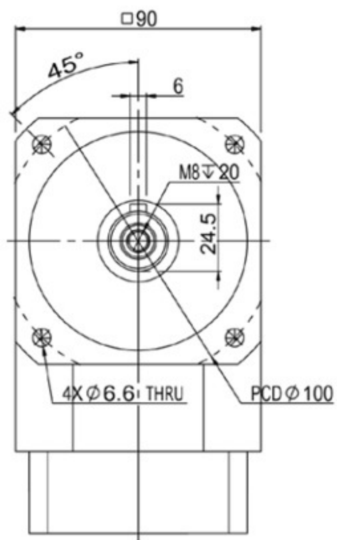
輸出端(output)
