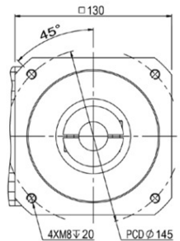
輸入端(input)
