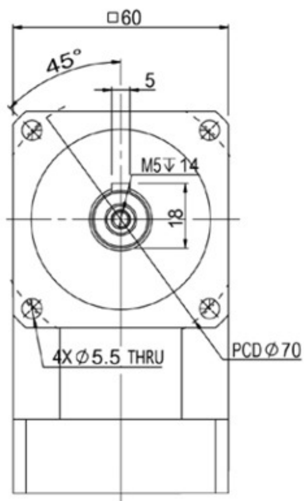
輸出端(output)
