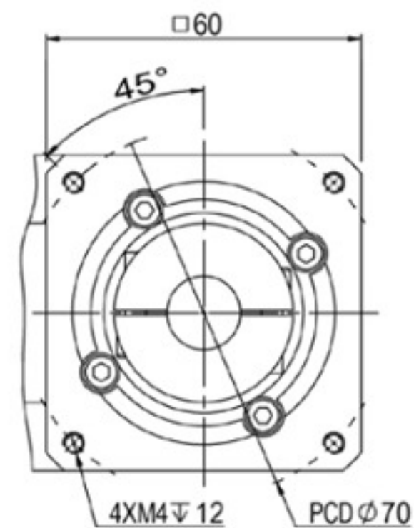
輸入端(input)
