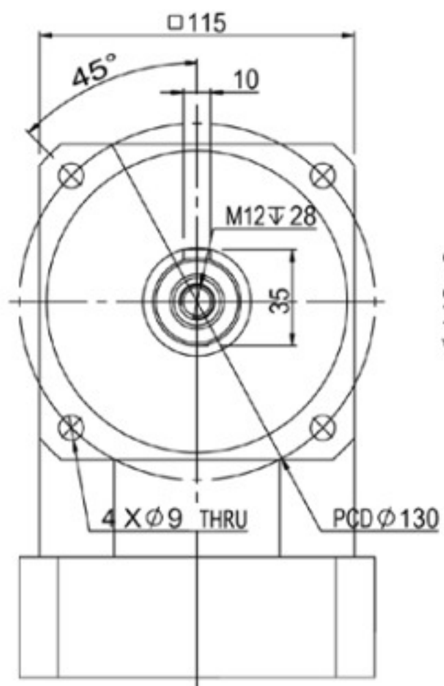
輸出端(output)
